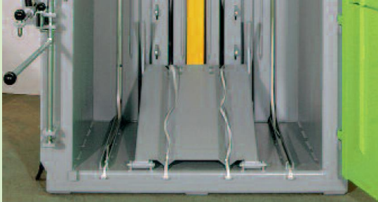
Der Auswerfer
